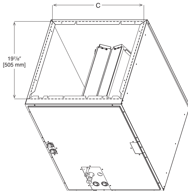
PLENUM WIDTH
